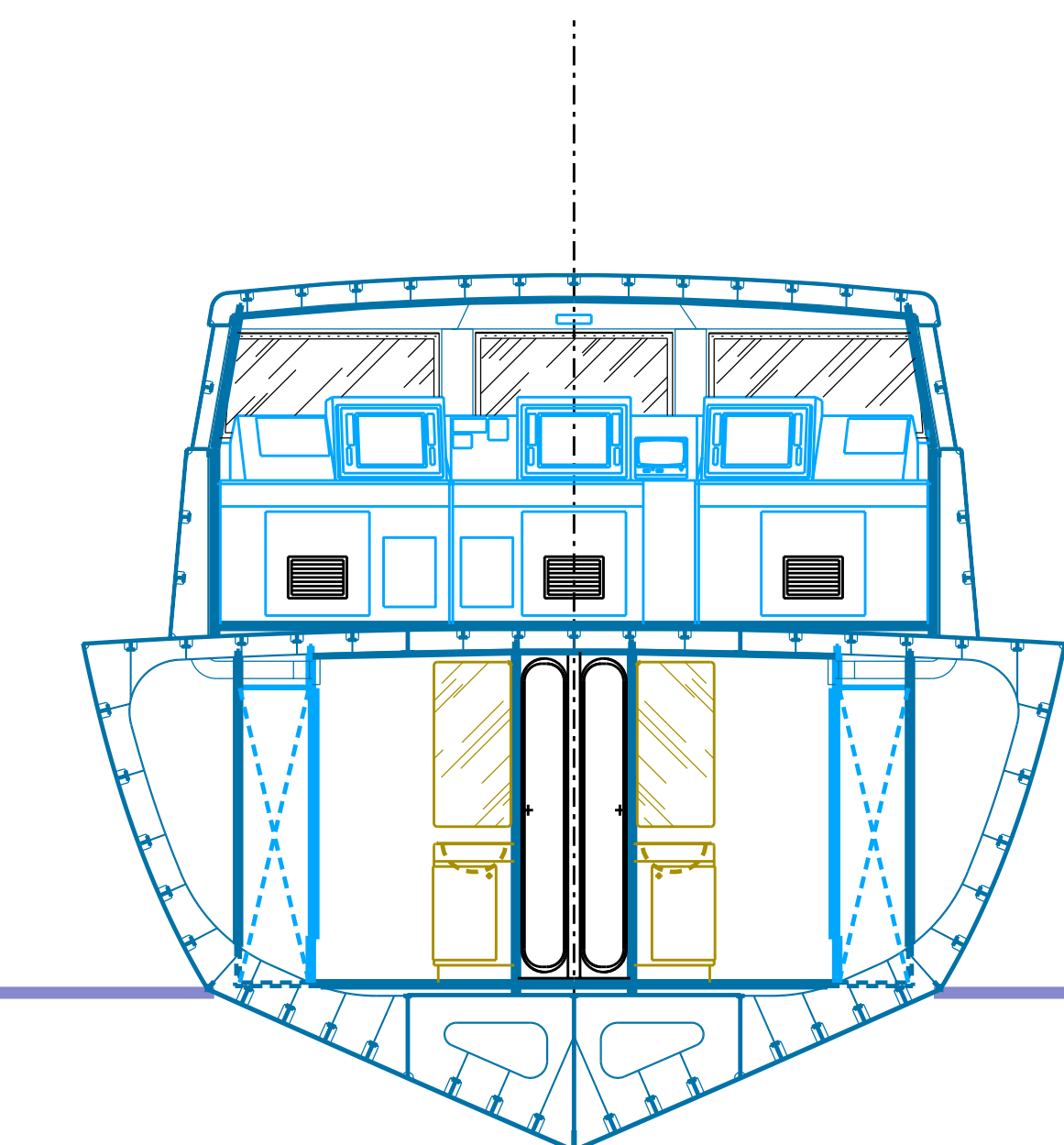
SEZIONE SU OSS. 17 (guardando prora)
