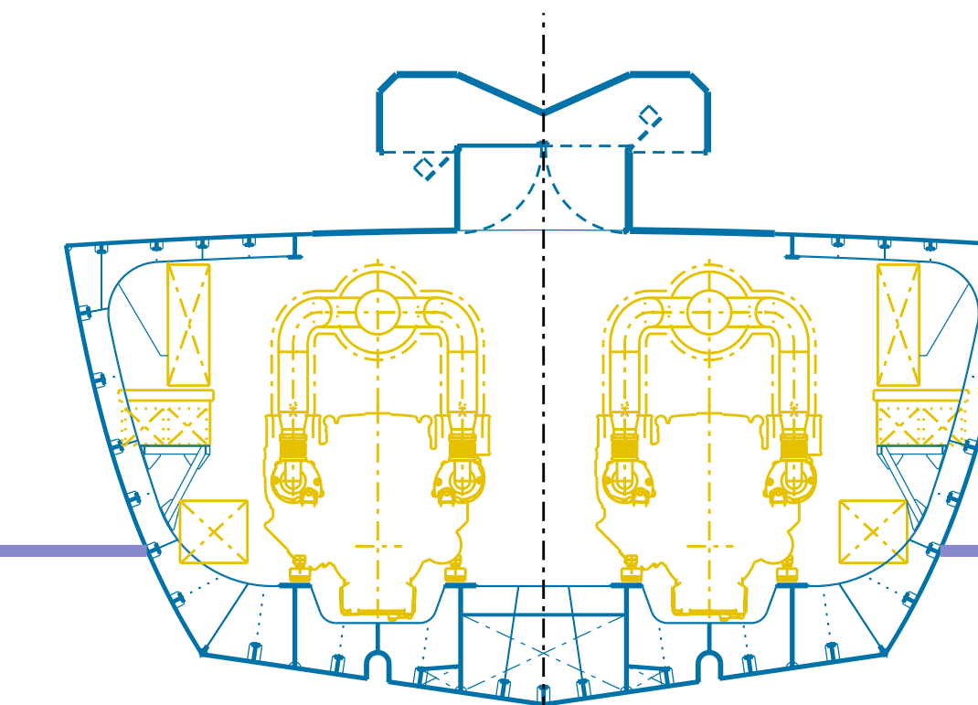
SEZIONE SU OSS. 5 (guardando prora)
