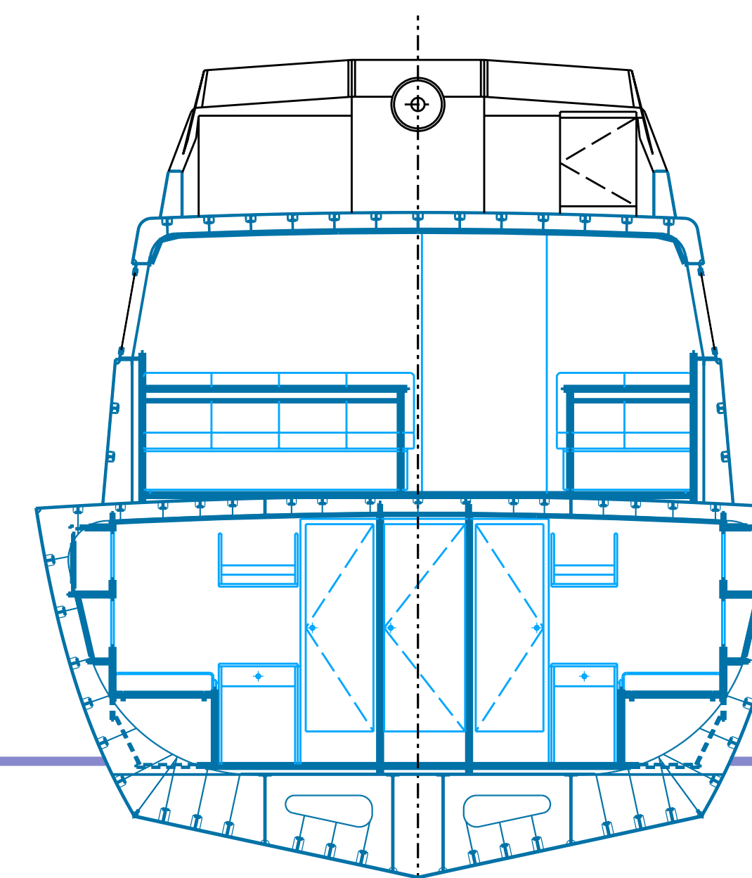
SEZIONE SU OSS. 12 (guardando prora)
