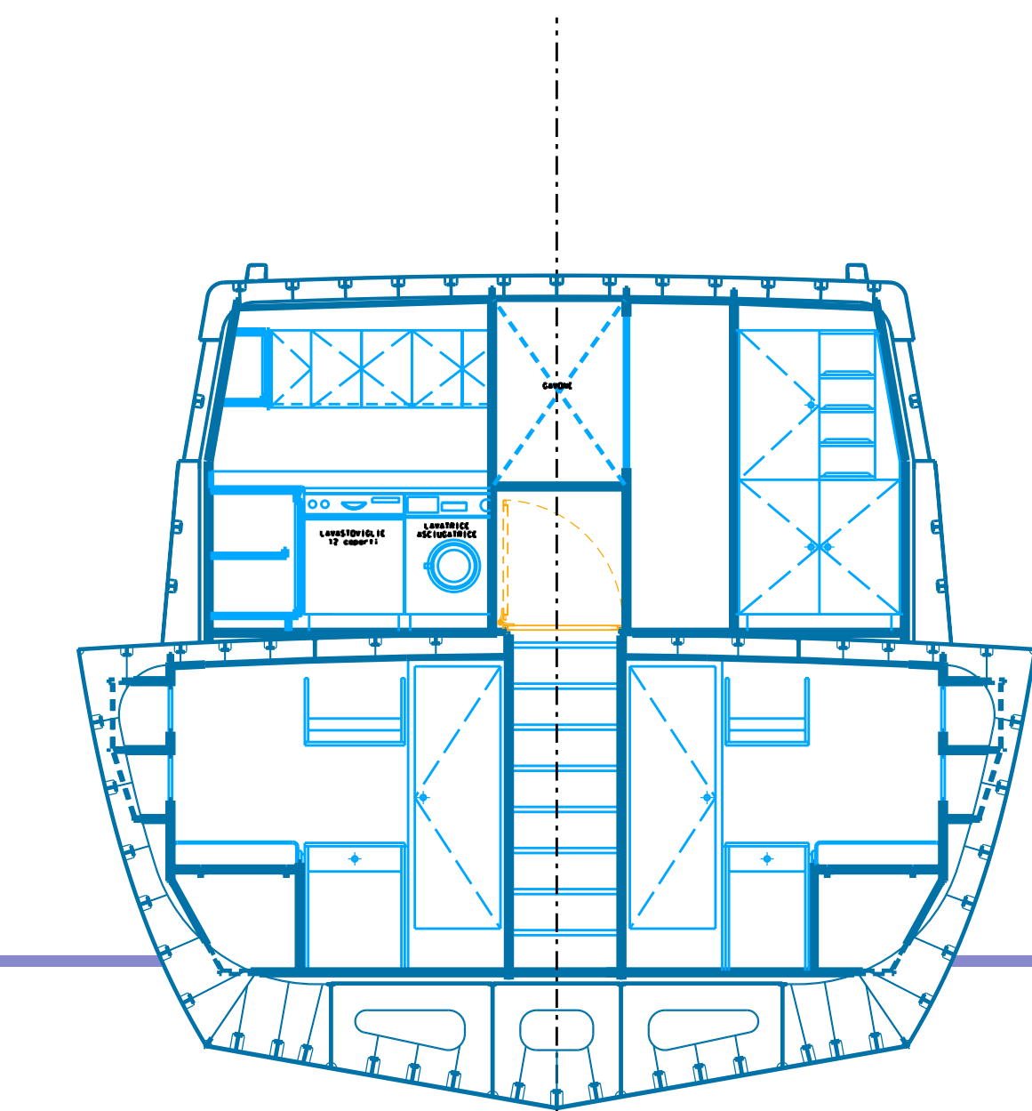
SEZIONE SU OSS. 10 (guardando prora)
